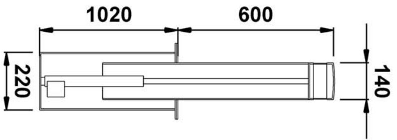
Automatischer Poller 60/14 AR
