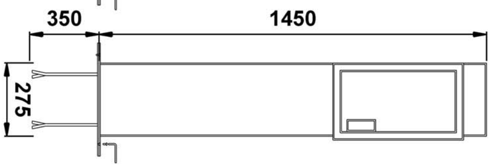
Poller Standsäule 275
