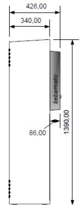
Seitenansicht Terminal Platinum Side view terminal Platinum
