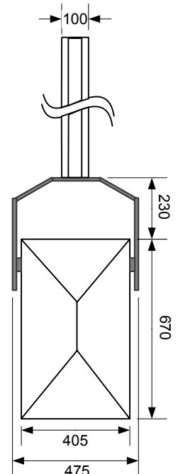
Draufsicht Top view
