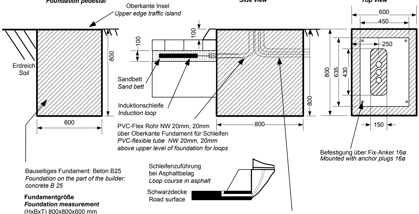
Seitenansicht Side view
