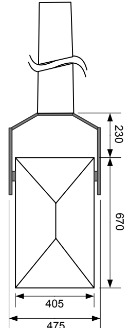
Draufsicht Top view
